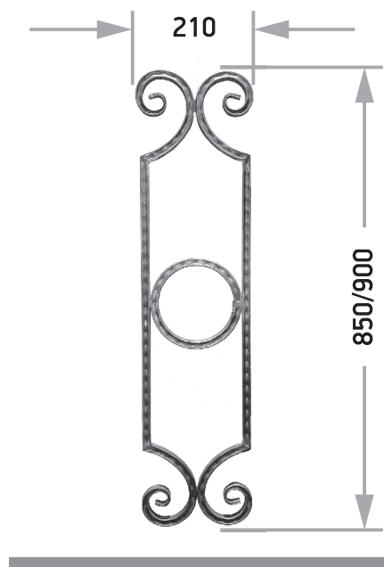
Артикул К 015 □15x15 Длина 850/900 Ширина 210
