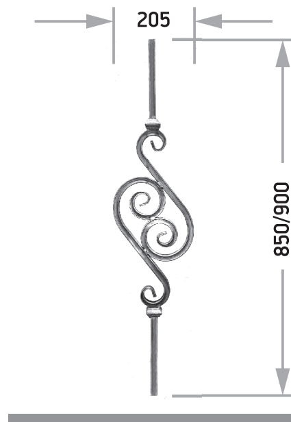
Артикул К 014 □15x15 Длина 850/900 Ширина 205
