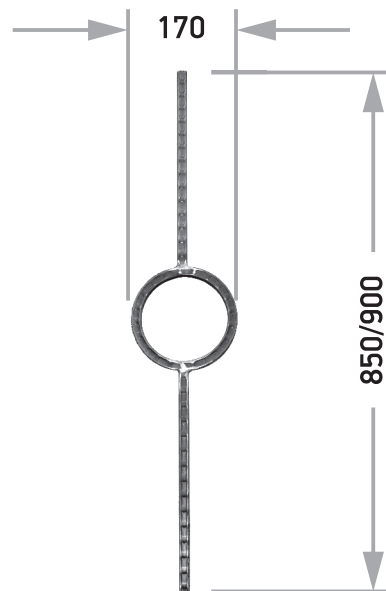
Артикул К 012 □15x15 Длина 850/900 Ширина 170
