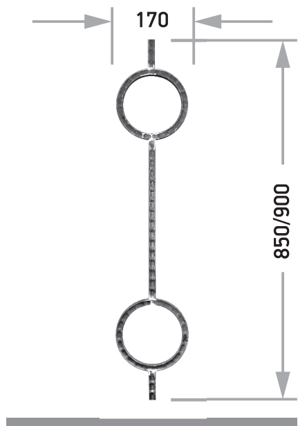
Артикул К 013 □15x15 Длина 850/900 Ширина 170
