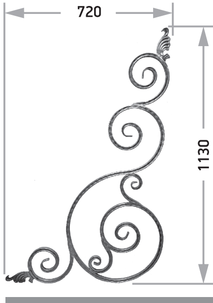
Артикул К 025 □15x15 Длина 1130 Ширина 720
