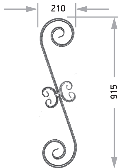
Артикул К 002 □15x15 Длина 915 Ширина 210
