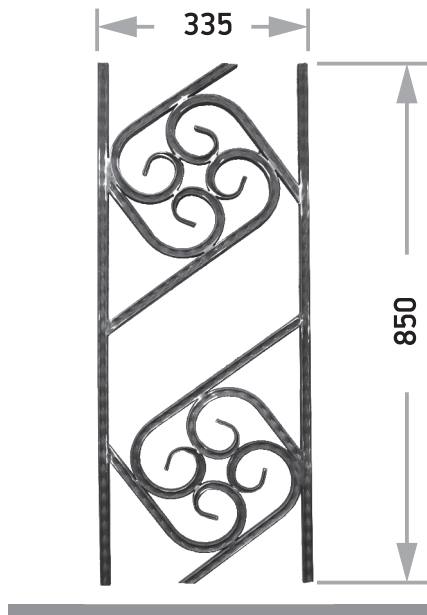
Артикул К 043 □15x15 Длина 850 Ширина 335
